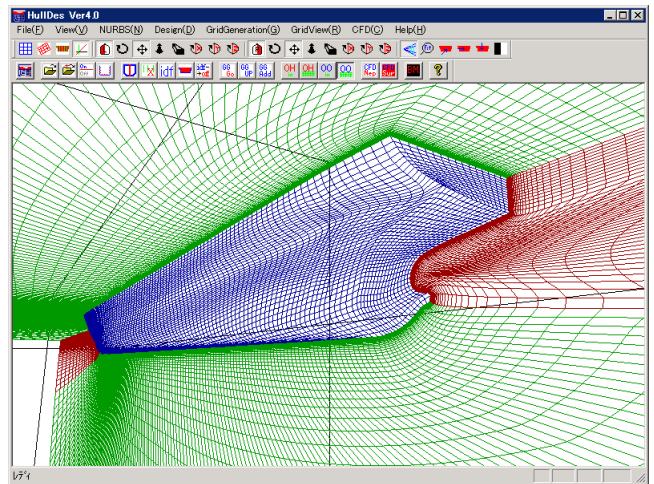
船体まわり格子作成例
