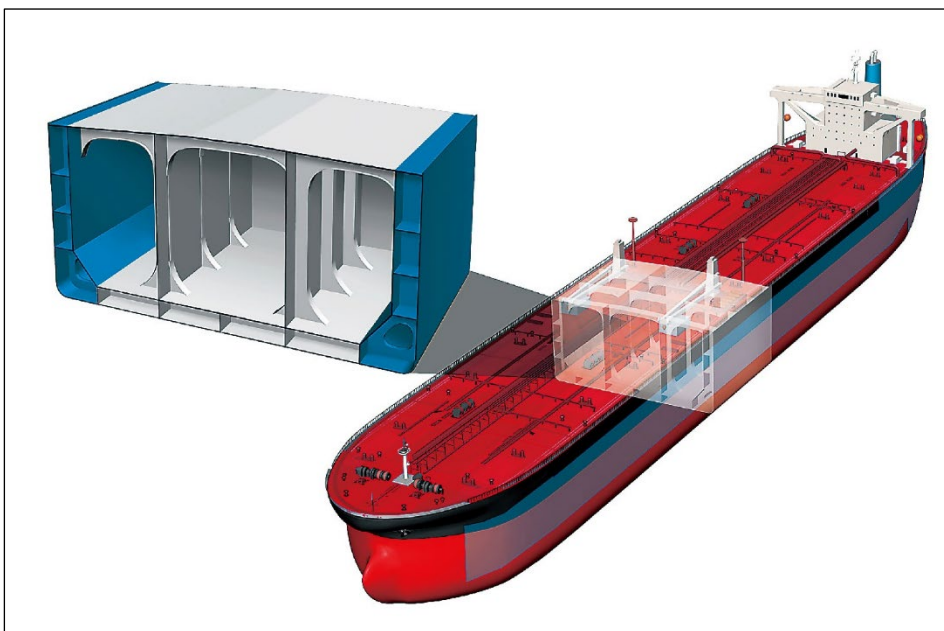
【図 2 超大型原油タンカーへの高延性厚鋼板の適用例】
