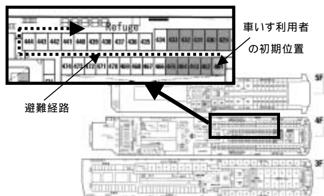
図-1 対象船一般配置図
