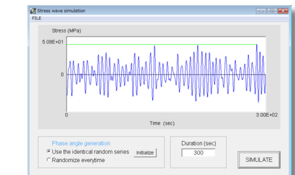
SPECTRUNの応力波形シミュレーション画面
