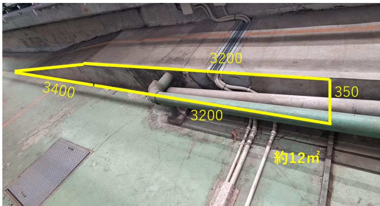
図 5 東西通路 西側通路部②
