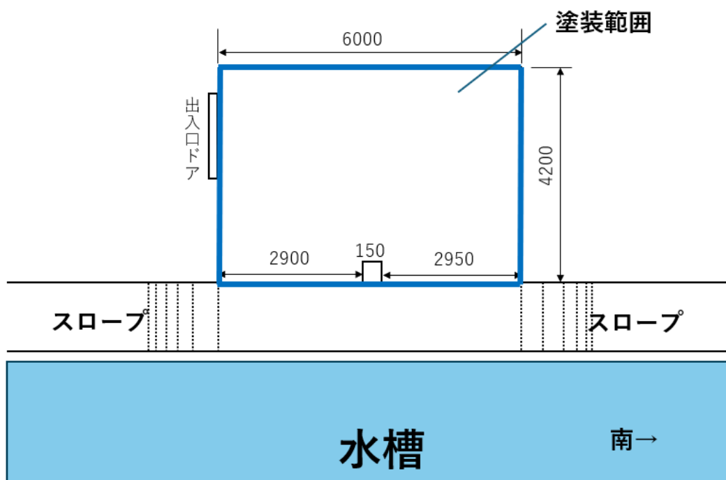
図 6 中間室 塗装範囲概略
