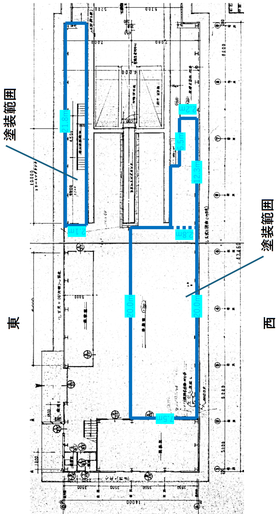
図1 準備場塗装箇所①
