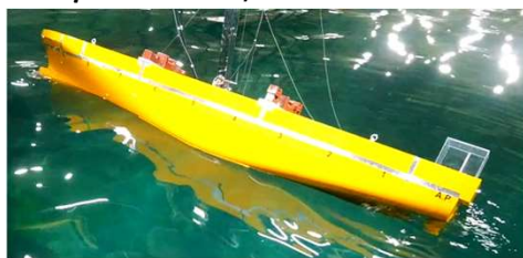
短波頂不規則波中のパラメトリック横揺れ
