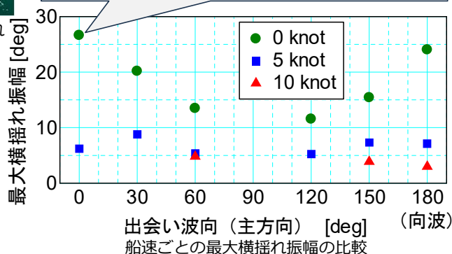
短波頂不規則波中のパラメトリック横揺れ
