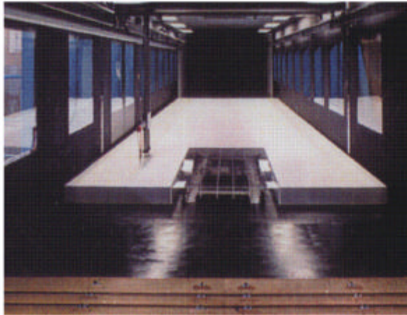
変動風水洞
