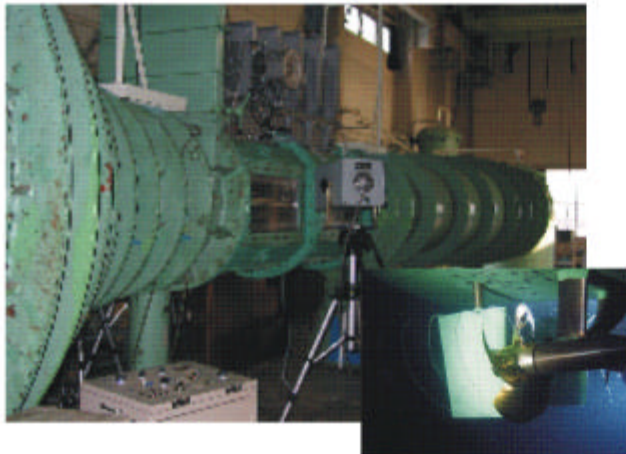
船尾変動圧計測 大型キャビテーション試験水槽
