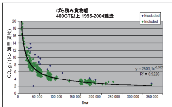
図-6 ばら積み貨物船 EEDI ベースライン例
