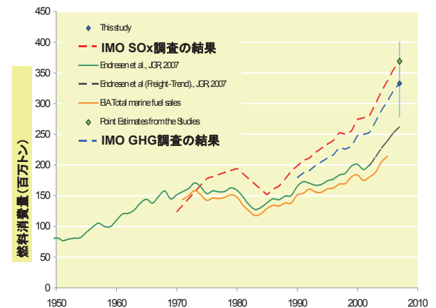
図-1 2007年までの国際航行船舶CO 2 排出算定
