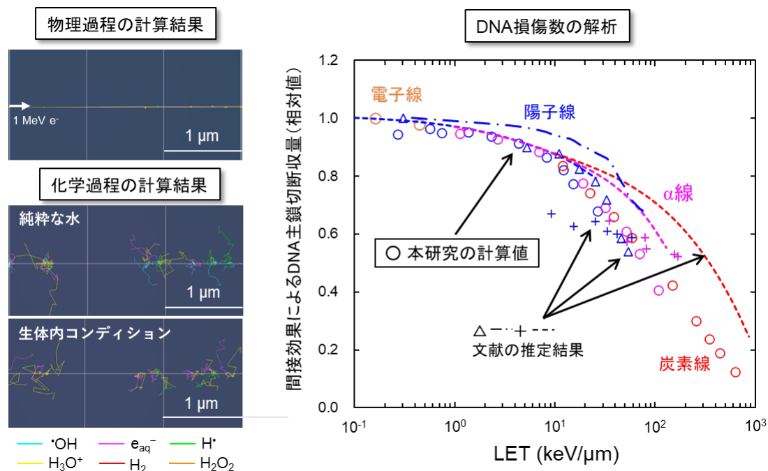
図 3 生命科学分野への応用として、DNA 主鎖切断 13) 数の解析を行いました。左上は 1\text{ MeV}^{14)} の電子線の飛跡、左中と左下は純粋な水中と生体内の分解生成物の挙動を追跡した結果です。右に、放射線の LET と間接効果の発生確率の関係を示します。
