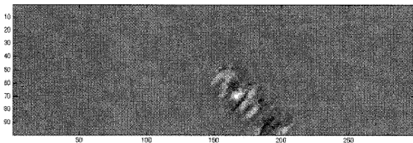
400-4 差分画像 亀裂高さ 2mm 画像-亀裂なし画像
