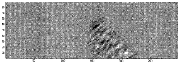
400-3 差分画像 亀裂高さ 8mm 画像-亀裂なし画像
