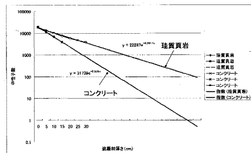
図2の近似線で外挿した珪質頁岩の中性子線遮蔽効果を示すグラフ図
