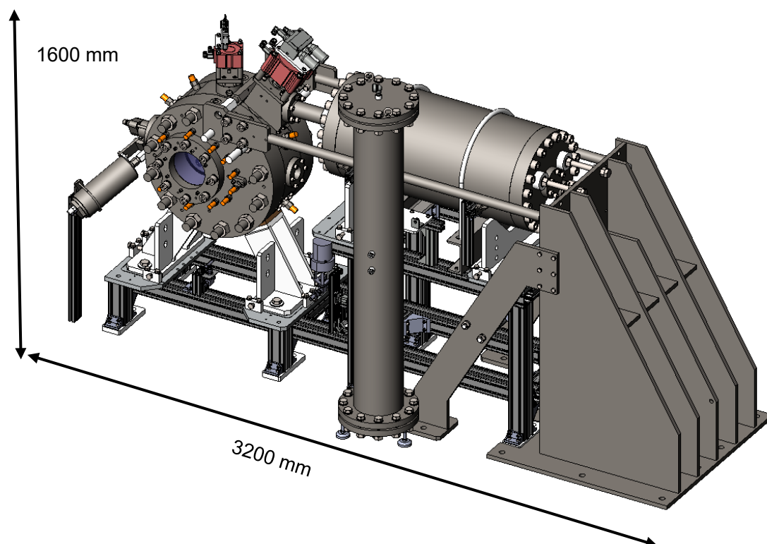
付図 1：燃焼試験装置の外観図
