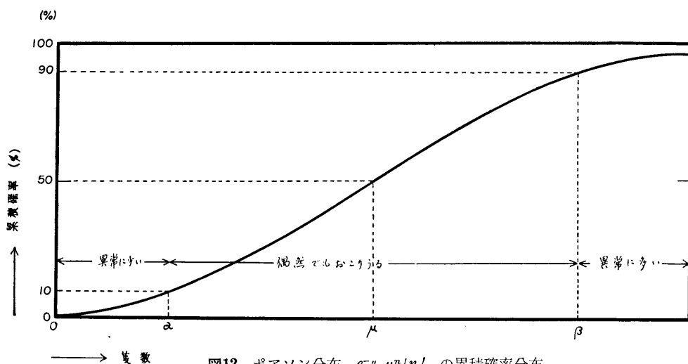
図12 ポアソン分布, e^{-\mu} \mu^n/n! , の累積確率分布
