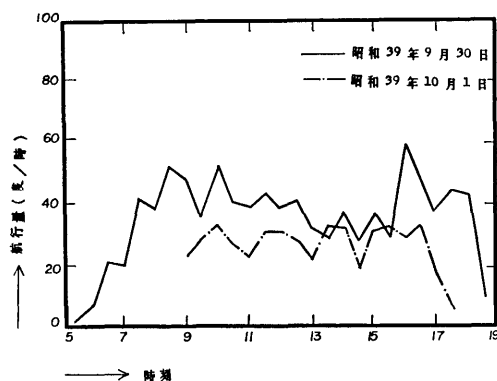
図5 横浜方面に向う船の航行量の時間変化
