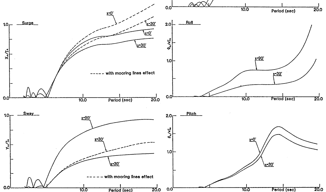
図-10 動揺の応答関数
