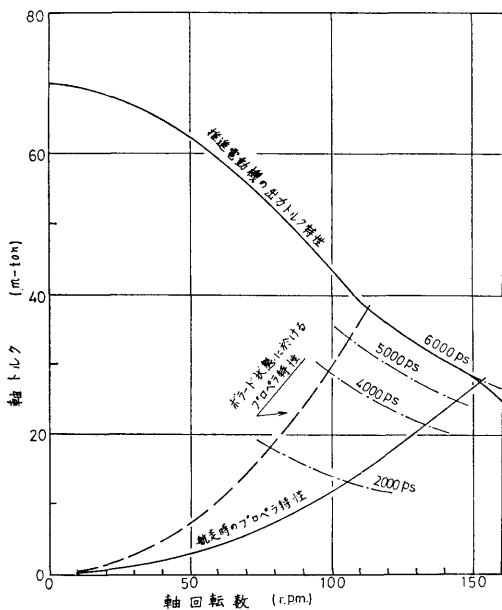
図-2.3 推進電動機速度-トルク特性曲線
