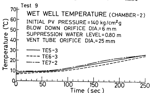
図 5-9 (e) No.9 実験のウェットウェル温度 (第2 圧力抑制室)
