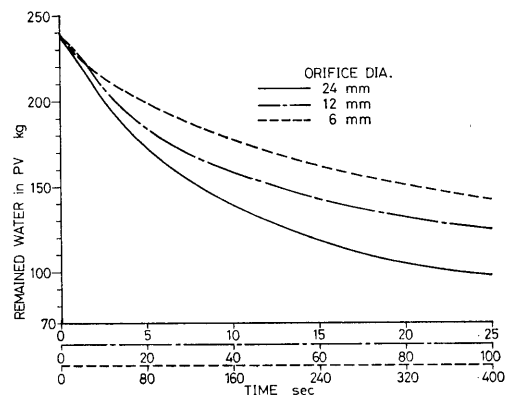
図 6-1 (b) 換算時間スケールによる压力容器内残留水の時間変化
