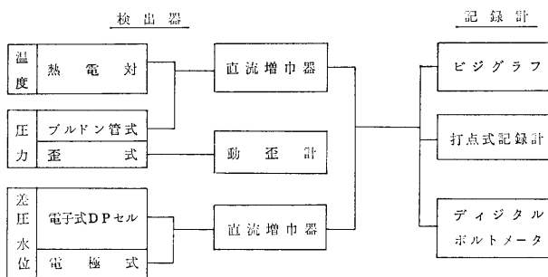
図 3-10 計装記録概念図
