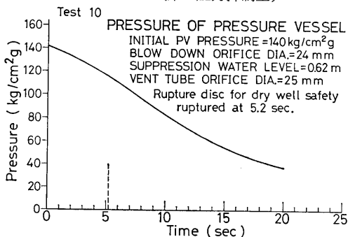
図 5-10 (a) No.10 実験の圧力容器内圧力
