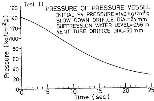
図 5-11 (a) No.11 実験の压力容器内圧力
