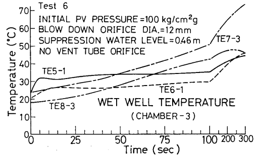
図 5-6 (e) No.6 実験のウェットウェル温度 (第3圧力抑制室)
