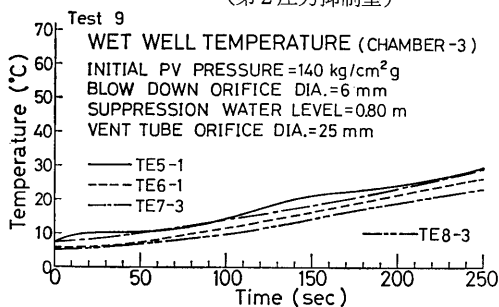
図 5-9 (f) No.9 実験のウェットウェル温度 (第3 圧力抑制室)
