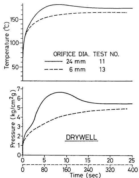
図 6-7 換算時間スケールによるドライウェル温度と圧力の比較
