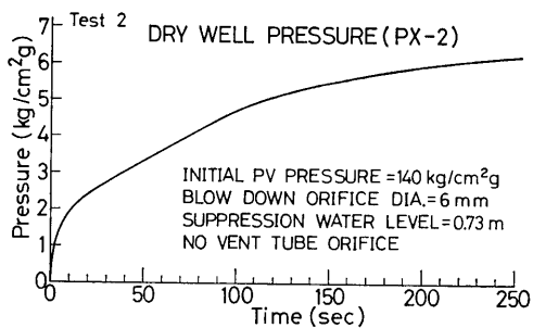
図 5-2 (b) No.2 実験のドライウェル圧力
