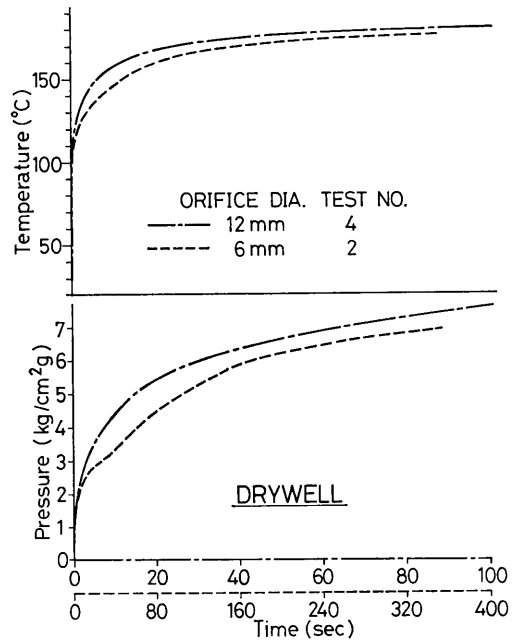
図6-4 換算時間スケールによるドライウェル温度と圧力の比較
