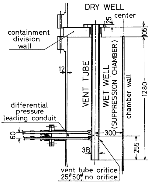
図 3-6 Vent Tube Details
