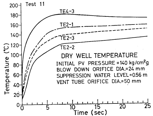
図 5-11 (d) No.11 実験のドライウェル温度
