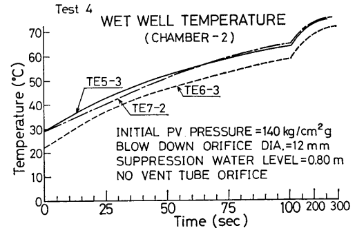
図 5-4 (d) No.4 実験のウェットウェル温度 (第2圧力抑制室)
