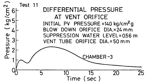
図 5-11 (c) No.11 実験のベント管オリフィス差圧
