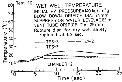
図 5-10 (e) No.10 実験のウェットウェル温度 (第2 圧力抑制室)
