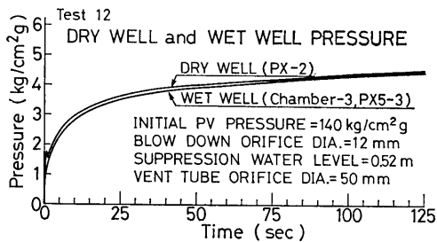
図 5-12 (b) No.12 実験のドライウェルとウェットウェルの圧力
