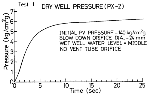
図 5-1 (b) No.1 実験のドライウェル圧力
