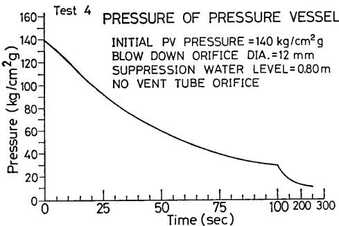
図 5-4 (a) No.4 実験の圧力容器内圧力
