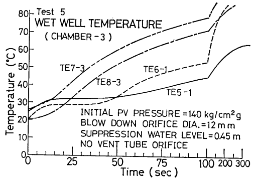
図 5-5 (e) No.5 実験のウェットウェル温度 (第3 圧力抑制室)
