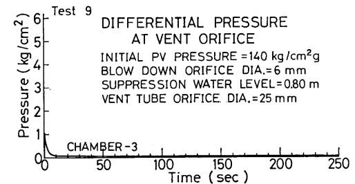
図 5-9 (c) No.9 実験のベント管オリフィス差圧
