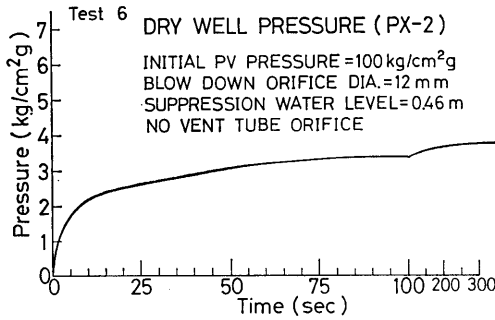
図 5-6 (b) No.6 実験のドライウェル圧力
