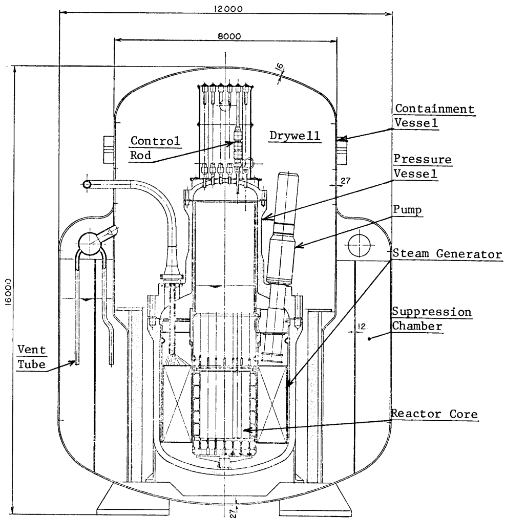
図 3-1 概念設計炉の格納容器構造図 (14)
