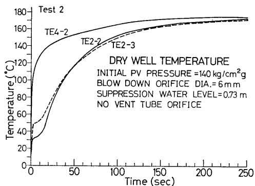
図 5-2 (c) No.2 実験のドライウェル温度
