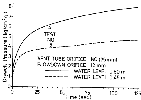
図6-2 ドライウェル圧力に対するウェットウェル水位の影響
