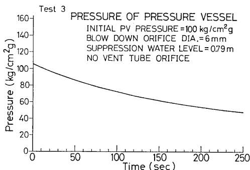
図 5-3 (a) No.3 実験の压力容器内圧力
