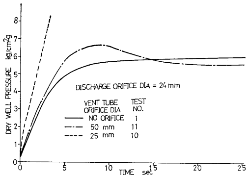
図 6-5 ドライウェル圧力に対するベント管絞りの影響
