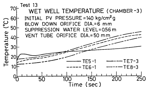
図 5-13 (e) No.13 実験のウェットウェル温度 (第3 圧力抑制室)
