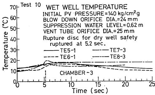
図 5-10 (f) No.10 実験のウェットウェル温度 (第3 圧力抑制室)
