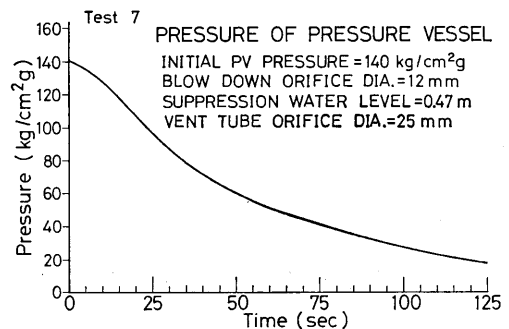
図 5-7 (a) No.7 実験の圧力容器内圧力
