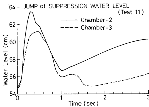
図 5-21 プールスウェルの測定例 (No.11実験)
