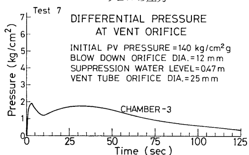
図 5-7 (c) No.7 実験のベント管オリフィス差圧
