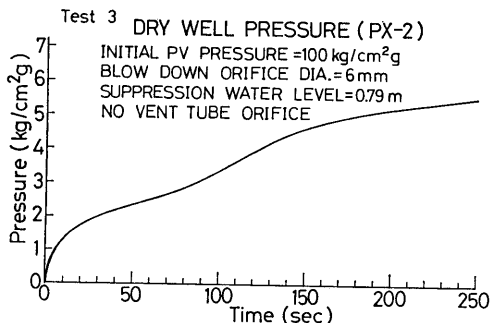
図 5-3 (b) No.3 実験のドライウェル圧力
