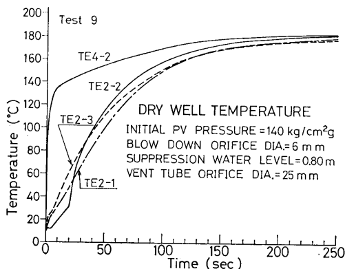
図 5-9 (d) No.9 実験のドライウェル温度
