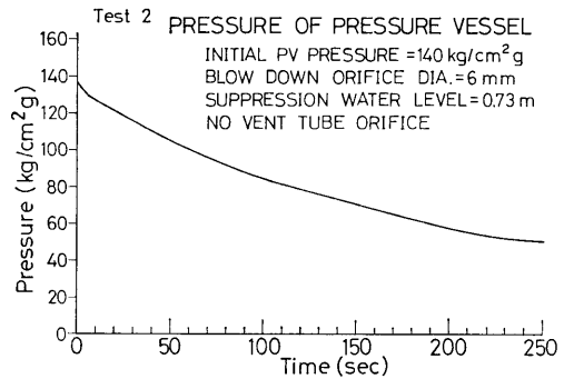
図 5-2 (a) No.2 実験の圧力容器内圧力
