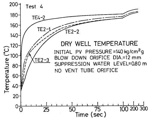
図 5-4 (c) No.4 実験のドライウェル温度
