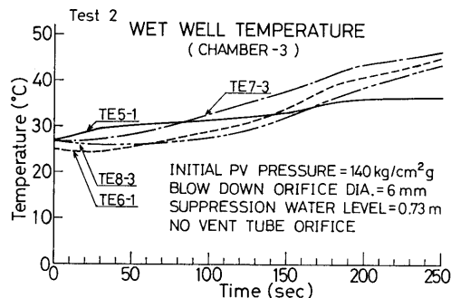
図 5-2 (e) No.2 実験のウェットウェル温度 (第3圧力抑制室)
