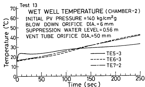
図 5-13 (d) No.13 実験のウェットウェル温度 (第2 圧力抑制室)
