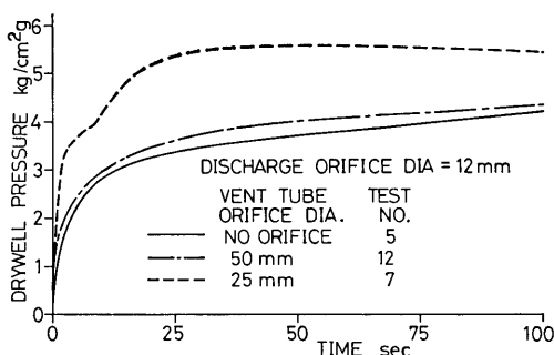
図 6-6 ドライウェル圧力に対するベント管絞りの影響
