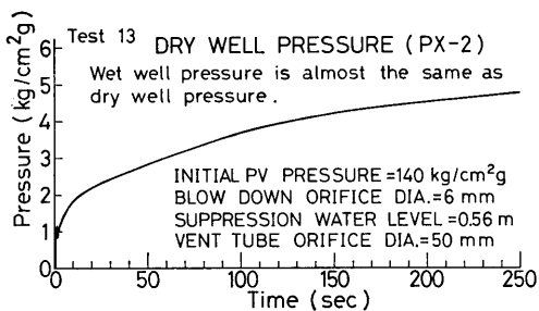
図 5-13 (b) No.13 実験のドライウェル圧力
