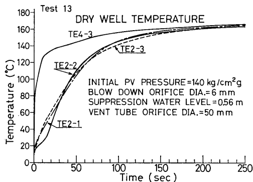
図 5-13 (c) No.13 実験のドライウェル温度
