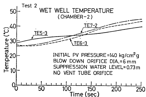
図 5-2 (d) No.2 実験のウェットウェル温度 (第2圧力抑制室)
