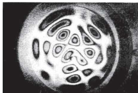
Fig. 6 ホログラフィによる振動パターンの観測例 6)
