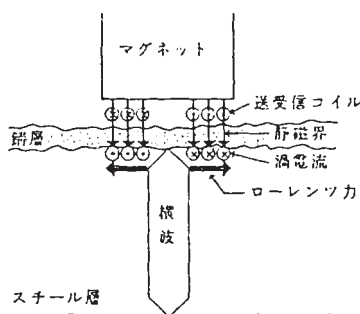
Fig.2 横波電磁超音波の原理 2)
