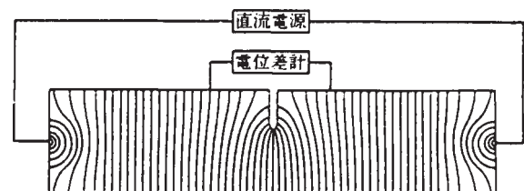
Fig.3 電気抵抗法の原理 3)
