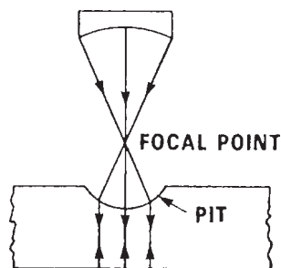
Fig.1 腐食部材に対する集束探触子の適用性 1)
