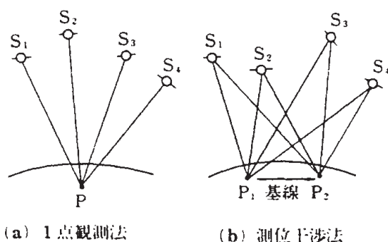
Fig.7 GPSによる測位 10)
