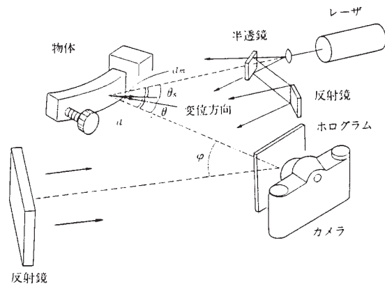
Fig. 5 ホログラフィの原理 5)
