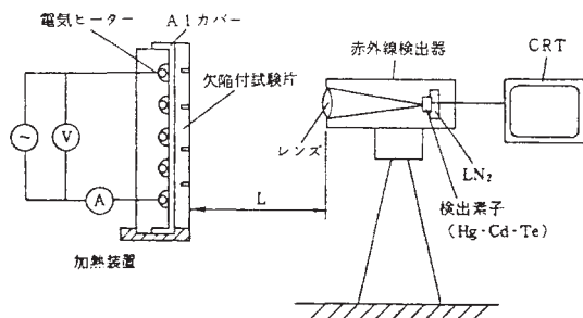
Fig. 4 サーモグラフィーによる欠陥検出 4)
