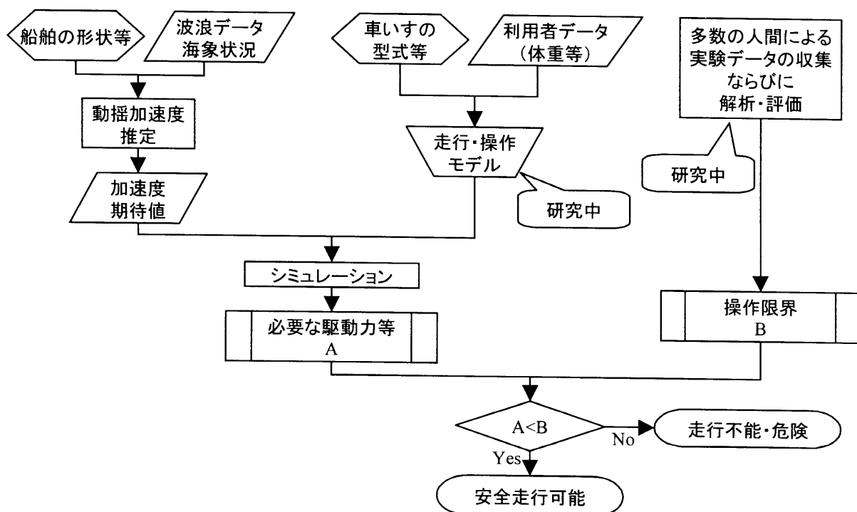
図－1 船内における車いすの自力走行限界の評価の流れ図
