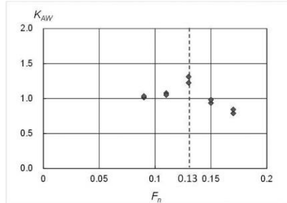
船速一波浪中抵抗増加の関係
